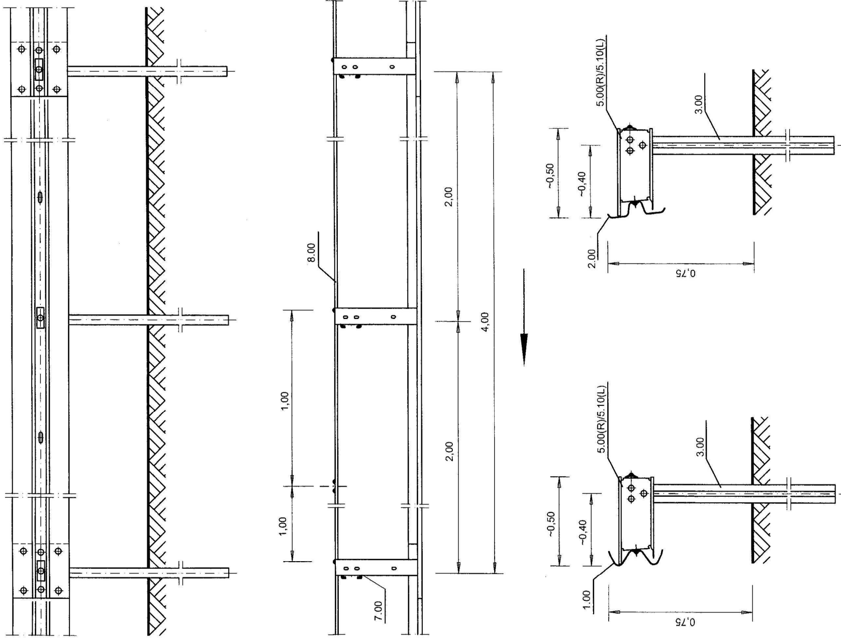
Verschraubung siehe Zeichnung Nr. B1.1-101
